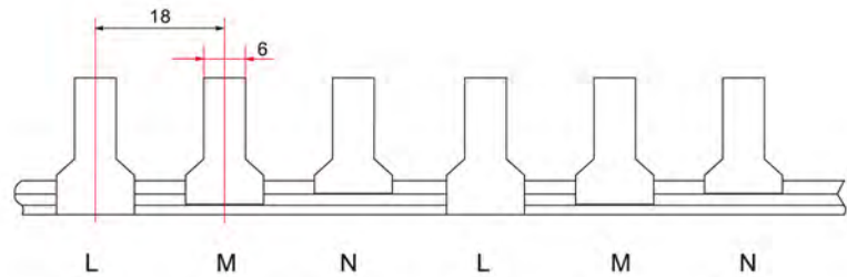
DZ47-3P
