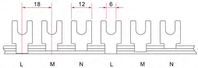
FBB-3P
