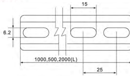
DG-001
