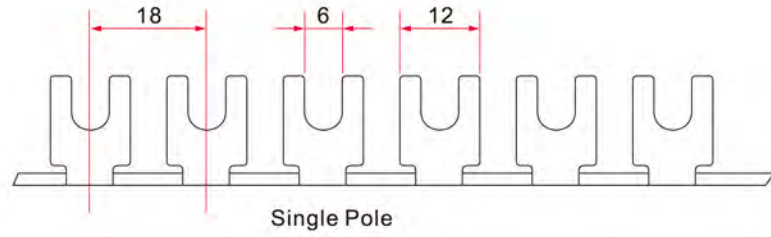
FBB-1P
