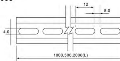
DG-003
