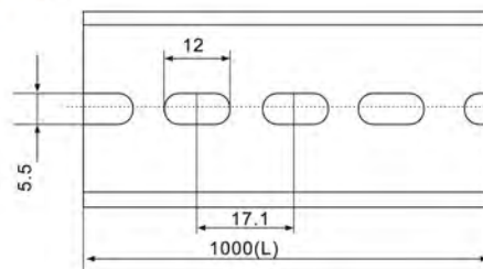
DL-011
