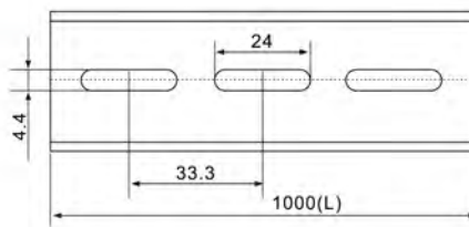
DL-012
